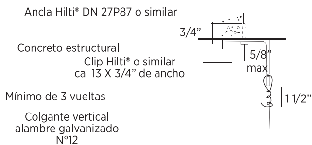
Detalle A Fijación Vertical de colgante
