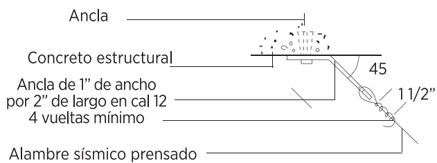
Detalle B Sujección lateral para poste de compresión
